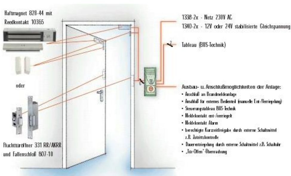
Systemdarstellung der Fluchttür-Verriegelung einer einflügeligen Fluchttür. Grafik und Fotos: Mink
