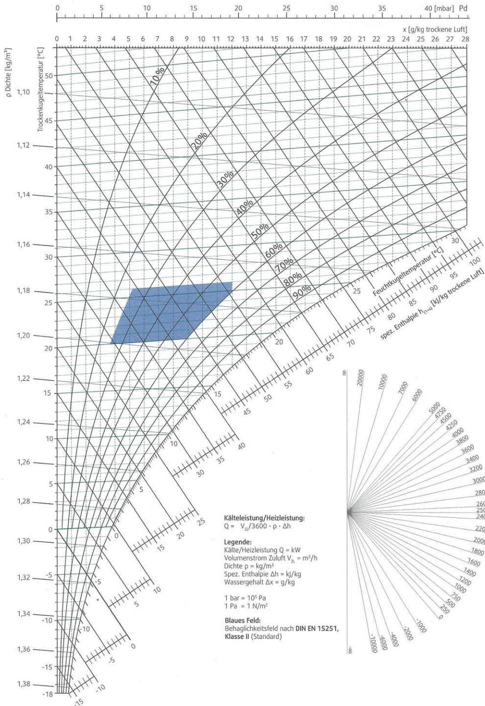
Mollier hx-Diagramm für 1,0133 bar
