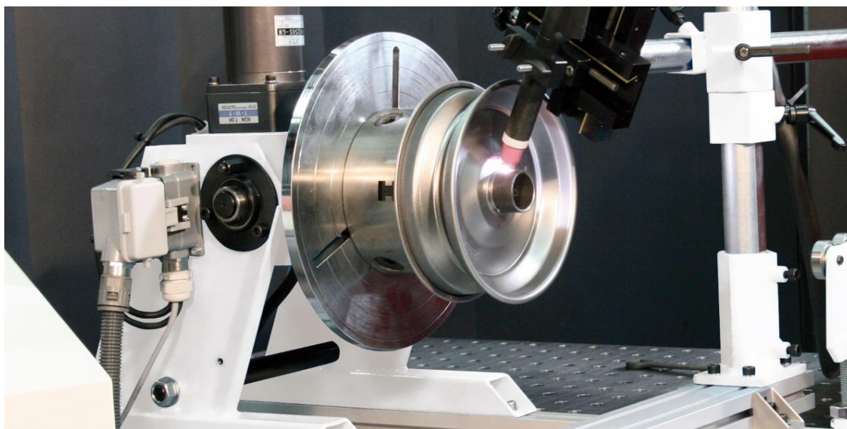
Positionierer mit Dreibackenfutter und Brennerstativ ermöglichen schnelles und vielseitiges Schweißen immer in der optimalen Position.
