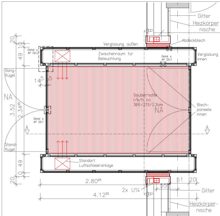
Planungsgrundriss.
