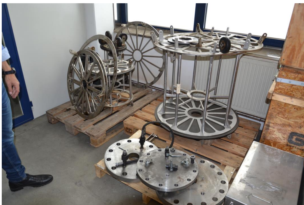
Die Fahrgestelle werden genau an die Anwendungsbedingungen angepasst.
