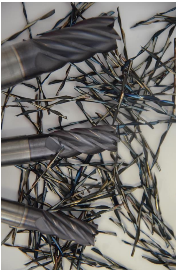
Die ungleiche Drallsteigung des Fräsers ermöglicht eine optimale Spanabfuhr.
