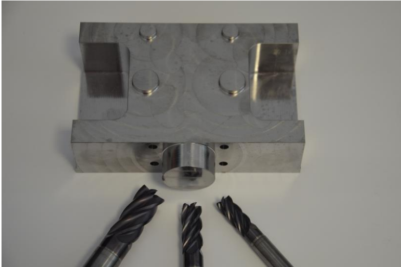
Gaden Konstruktion und Prototypenbau bearbeitet mit dem HAM-Fräser 40-5091 ein Bauteil aus Werkzeugstahl.
