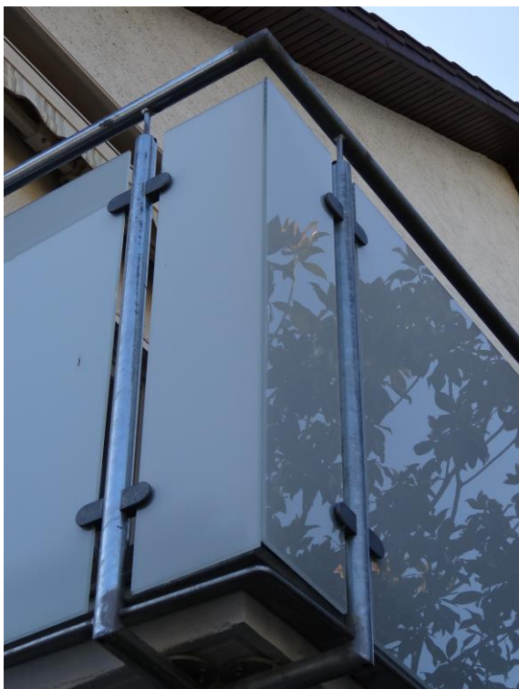
Die jeweiligen Scheiben zur Geländerecke sind nur mit zwei Glas-Randklemmhaltern abgesichert. Fotos: Sternberger
