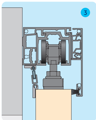
3. Wandmontage mit Variante A-B innen geklebt
