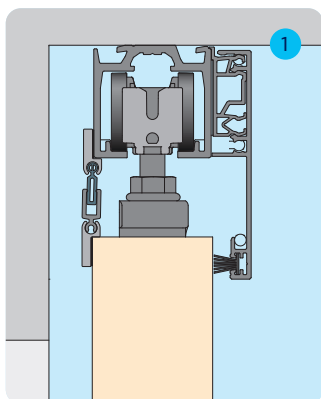
1. Deckenmontage Variante A-B
