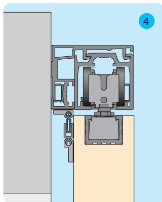
4. Wandmontage mit Variante A-B aussen geklebt
